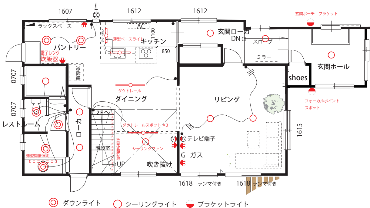
A 棟 電気配線計画
