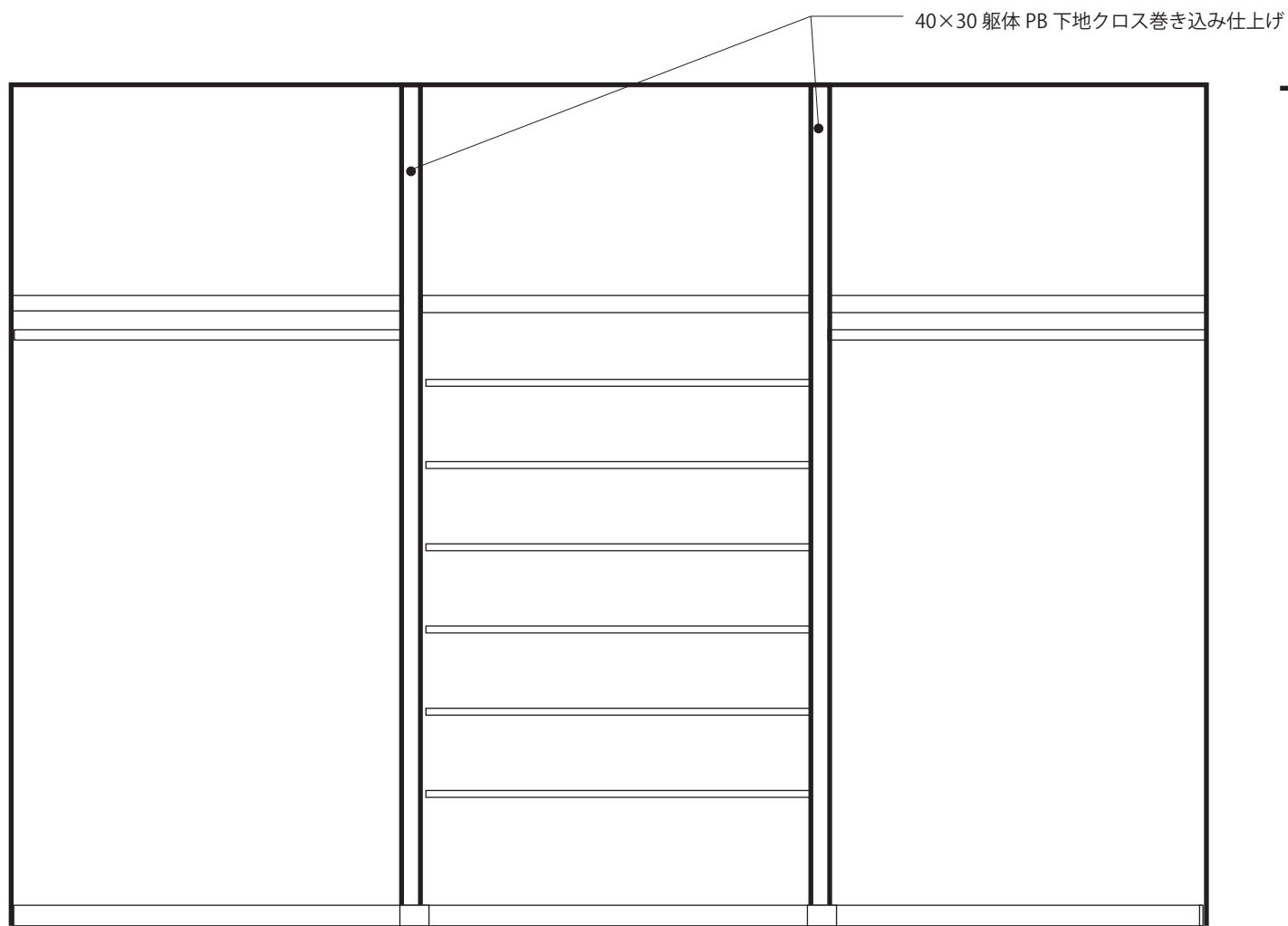
北・南面 エレベーション
