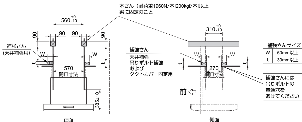
【参考値】 天吊ボルト、座金サイズ
